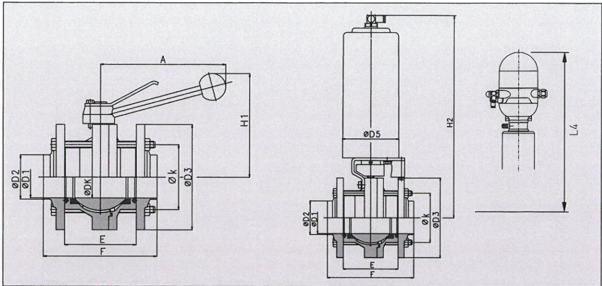
H 587 manually operated / handbetätigt
